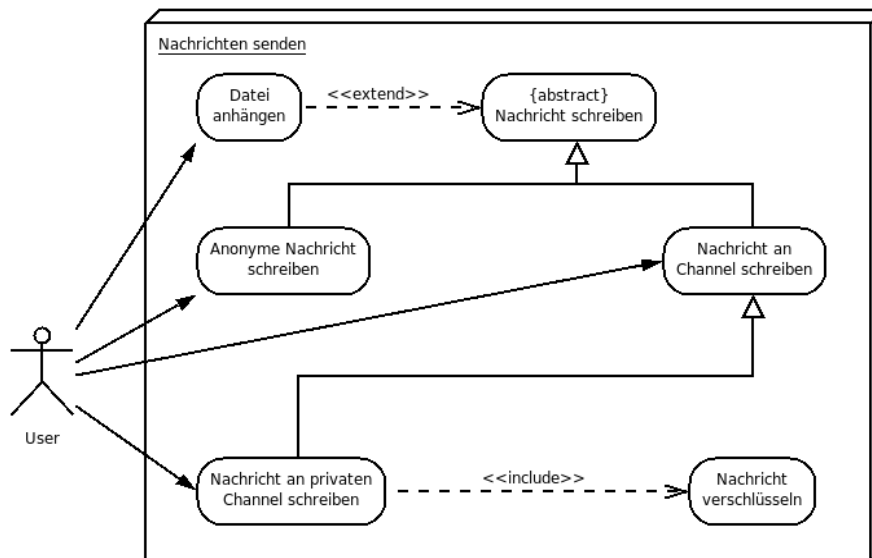
Abbildung 1: Use Case 1: Senden
