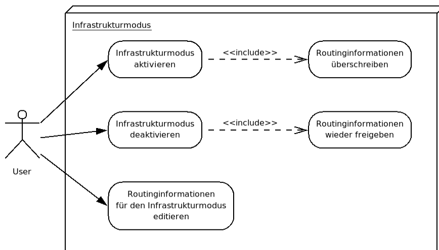
Abbildung 2: Use Case 2: Kanäle
